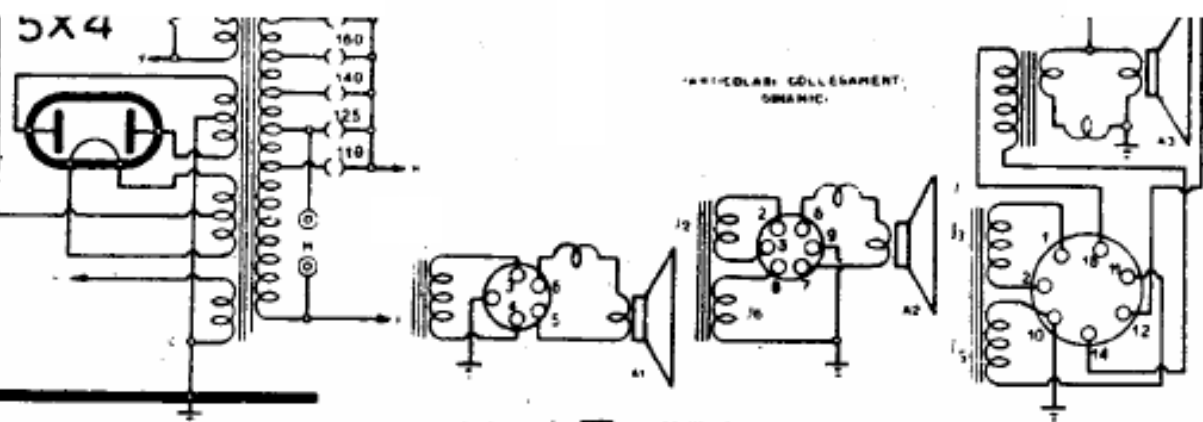
Questi due circuiti si accordano con il modello « IF 71 » III serie di cui è stato riprodotto lo schema
