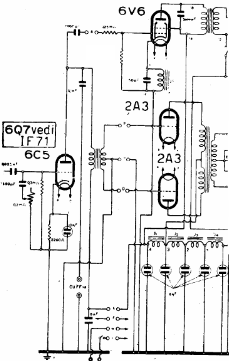
Questi due circuiti si accordano con il modello « IF 71 » III serie di cui è stato riprodotto lo schema
